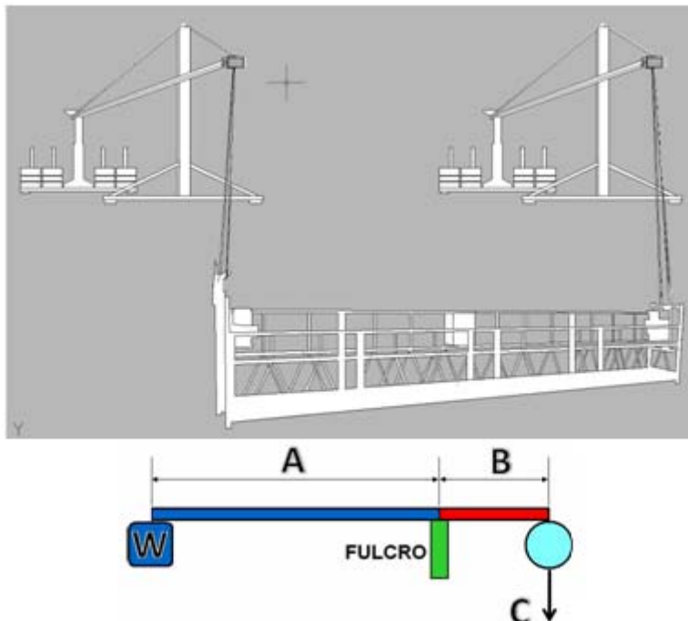
Figura 7 Contrapesos en andamios suspendidos
